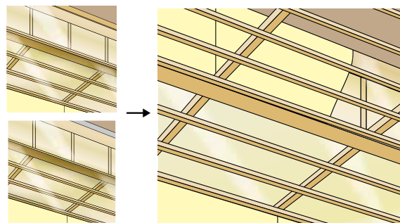
⑤天井野縁延長
