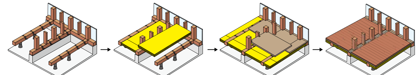
① 床用断熱材専用支持金物設置
